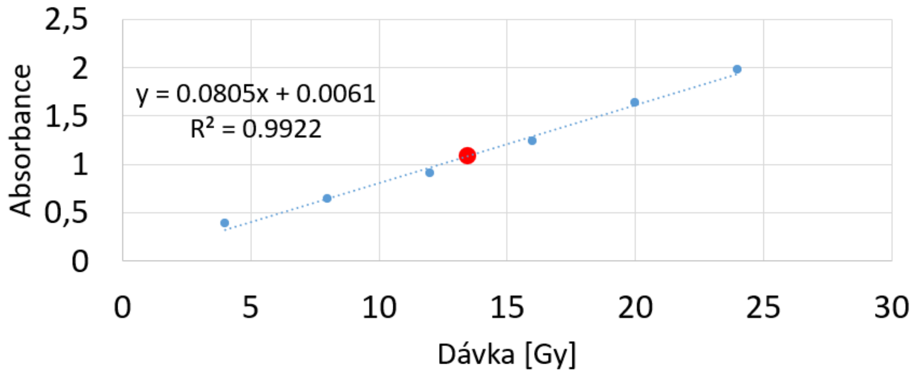
Kalibrační křivka
